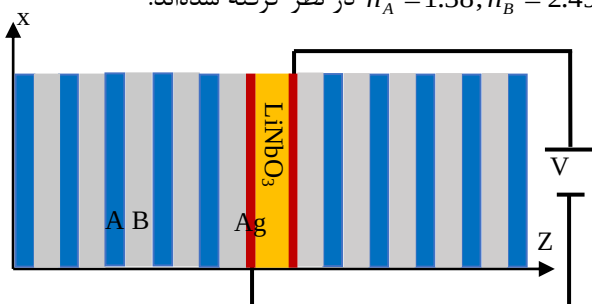
شکل ۱: شمایی از بلور فوتونی یک‌بعدی پیشنهادی برای طراحی کلید نوری به شکل (AB)^5 Ag LiNbO_3 Ag (BA)^5 . لیتیم نیوبات و دو لایه‌ی نقره، لایه‌های نقص ساختار متقارنند.
