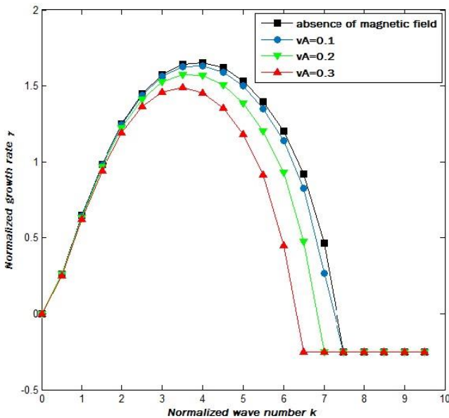
شکل ۲. نرخ رشد در مقایسه با عدد موج برای مقادیر مختلف از میدان مغناطیسی
