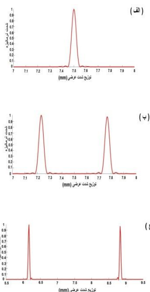
شکل ۳: نمودارهای توزیع شدت عرضی شبیه سازی شده در راستای z : الف) ( m=n=0 )، ب) ( m=0/5, n=0 ) و ج) ( m=2/5, n=0 ).
