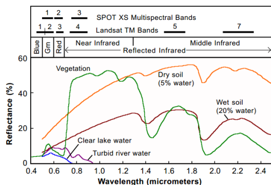
شکل ۱: نمونه‌ای از امضای طیفی مواد مختلف [۱]
