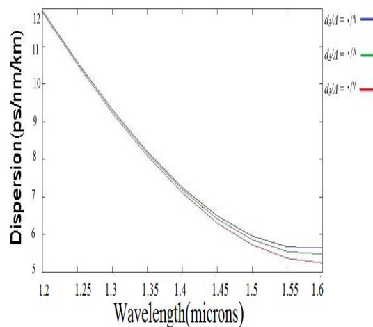
شکل ۵- اثر تغییر قطر حفره های سومین حلقه هوایی اطراف هسته بر میزان پاشندگی تار با در نظر گرفتن d_1/L = 0.18 و d_2/L = 0.17
