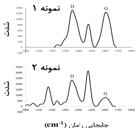
جایجایی رامان ( \text{cm}^{-1} )
