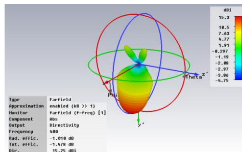
شکل ۶- الگوی تشعشعی آنتن پلاسمونی با ساختار ENZ تحقق یافته با استفاده از نانوکامپوزیتهای فلزی.
