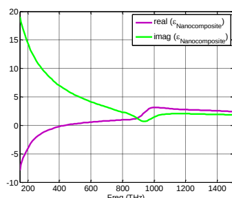
شکل ۱- قسمتهای حقیقی و موهومی ثابت دی‌الکتريک نانوکامپوزیت نقره در آلومینا.
