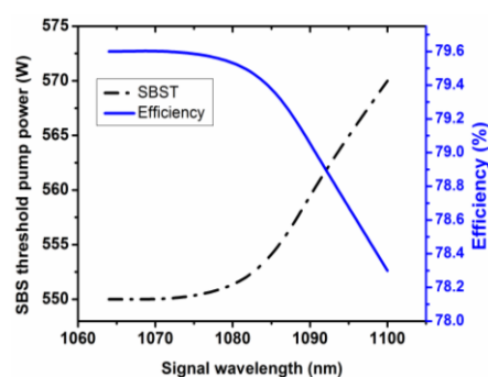
شکل ۳: تغییرات SBST و بازده بر حسب طول موج سیگنال خروجی
