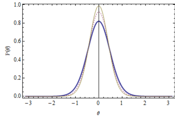
شکل ۲: تابع توزیع فاز پگ-بارنت حالت‌های همدوس فوتون‌افزوده‌ی نوسانگر ناهماهنگ برحسب \theta به ازای m=2 (خط توپر ضخیم)، m=5 (خط چین) و m=8 (خط توپر باریک).
