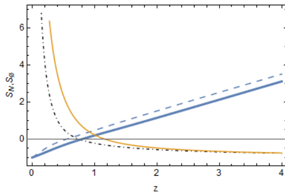
شکل ۳: چلانگی تعداد- فاز حالت‌های همدوس فوتون‌افزوده‌ی نوسانگر ناهماهنگ برحسب z به ازای m=1 \{S_N\} (خط توپر ضخیم)، S_\phi (خط توپر باریک) و m=3 \{S_N\} (خط چین)، S_\phi (نقطه خط چین)
