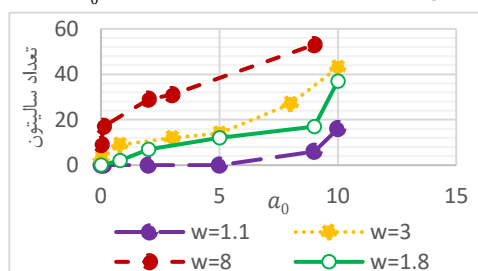
شکل ۷: بررسی تغییرات تعداد سالیتون بر حسب a_0
