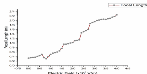
شکل ۴: نمودار تغییرات فاصله‌ی قانونی با تغییر میدان الکتریکی.
