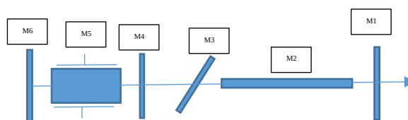
شکل ۵: چیدمان آزمایشگاهی برپا شده (در این چیدمان M1 آینه خروجی، M2 ماده فعال Nd:YAG، M3 پلاریزور، M4 تیغه چارک موجی، M5 سلول پاکلز، M6 آینه پشتی لیزر می‌باشد).
