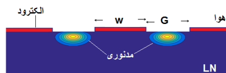
شکل ۲: مد نور موجبر با عرض ماسک 6\mu\text{m} با تبادل پرتون یک ساعت در دمای ۱۷۰ درجه و آنیل ۵ ساعت در دمای ۳۷۵ درجه در طول موج ۱۵۵۰ nm.
