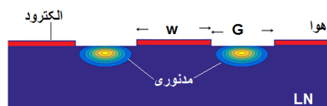
شکل ۲: مد نور موجبر با عرض ماسک ۶ μm با تبادل پروتون یک ساعت در دمای ۱۷۰ درجه و آنیل ۵ ساعت در دمای ۳۷۵ درجه در طول موج ۱۵۵۰ nm.
