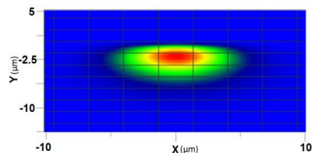
شکل ۲: مد نور موجبر با عرض ماسک ۶ μm با تبادل پروتون یک ساعت در دمای ۱۷۰ درجه و آنیل ۵ ساعت در دمای ۳۷۵ درجه در طول موج ۱۵۵۰ nm.
