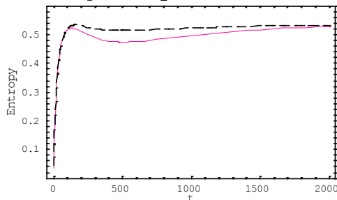
۴) کاهش آنتروپی \Omega_1 = .001 \Omega_2 = .0003 \gamma = .001 n = 5 در نمودارهای بالا \Omega_1, \Omega_2 ثابت‌های جفت شدگی مؤثر اتم-میدان در حضور و عدم حضور میدان لیزر خارجی هستند. n بیانگر تعداد فوتون‌های حرارتی و \gamma ثابت جفت شدگی سامانه با اتلافگر است.
