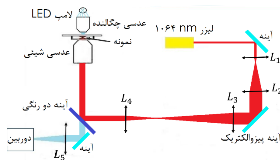
شکل ۳: چیدمان انبرک نوری چندتله‌ای.
