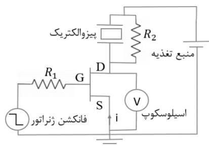
شکل ۴: طرح‌واره‌ای از مدار تغذیه بین‌الکترونیک توسط ماسفت.
