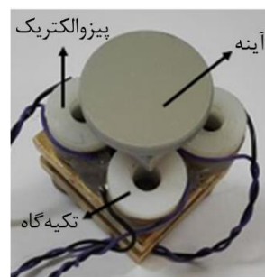
شکل ۲: تصویر مربوط به آینه پیزوالکتریک است.
