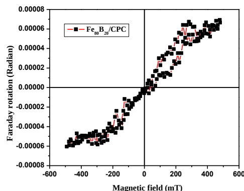
شکل ۵ - نمودار تغییرات شدت FR در دمای اتاق از نمونه \text{Fe}_x\text{B}_{20}/\text{CPC}
