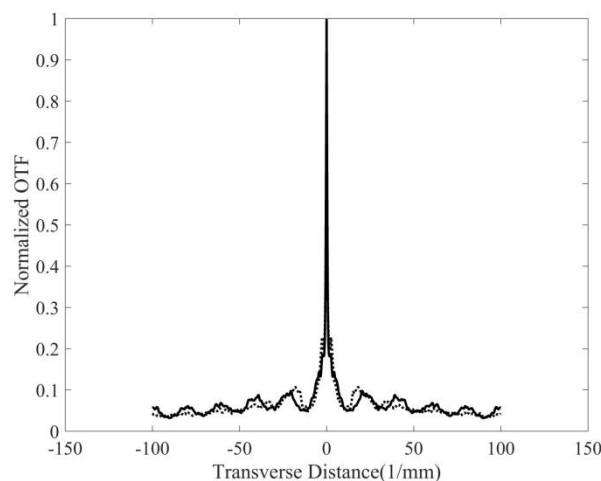
شکل ۳: تابع انتقال اپتیکی بهنجار، خط ممتد برای \alpha=8 و نقطه‌چین
