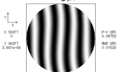
شکل ۸: الگوی تداخلی در نتیجه‌ی اعمال خطا به میزان 0.008333'' = 30\text{arcsec} در هم‌مرکزی عدسی جبران کننده
