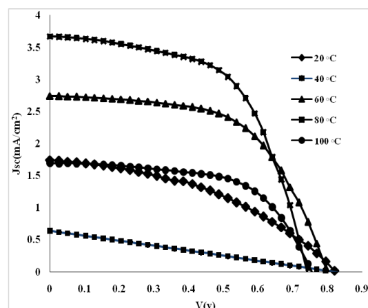
شکل ۱: نمودار چگالی جریان-ولتاژ مربوط به دماهای مختلف غوطه‌وری.
