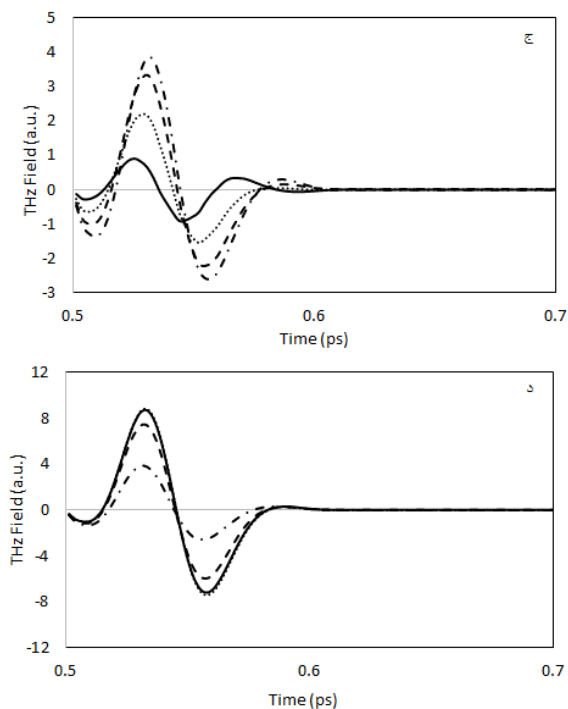
شکل ۴: میدان تراهرتز (الف) در فشار ۱۰۰ (نقطه‌چین) و ۴۰۰ torr (خط‌چین) و ۱ atm (خط توپر) در گاز نیتروژن؛ (ب) در گازهای زمینه‌ی هلیوم (نقطه‌چین)، نئون (خط‌چین) و آرگون (خط توپر) در فشار ۱ atm؛ (ج) به ازای اختلاف فازهای ۰ (خط توپر)، ۳۰ (نقطه‌چین)، ۶۰ (خط‌چین) و ۹۰° (خط نقطه) در فاز اولیه‌ی ثابت صفر و (د) به ازای فازهای اولیه‌ی ۰ (خط نقطه)، ۳۰ (خط‌چین)، ۶۰ (خط توپر) و ۹۰° (نقطه‌چین) در اختلاف فاز ۹۰°.
