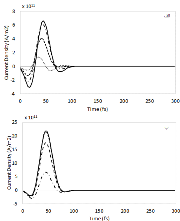
شکل ۳: توزیع زمانی چگالی جریان عرضی خالص (الف) به ازای اختلاف فازهای ۰ (نقطه‌چین)، ۳۰ (خط‌چین)، ۶۰ (خط نقطه) و ۹۰° (خط توپر) در فاز اولیه‌ی ثابت صفر و (ب) به ازای فازهای اولیه‌ی ۰ (خط نقطه)، ۳۰ (خط‌چین)، ۶۰ (نقطه‌چین) و ۹۰° (خط توپر) در اختلاف فاز ثابت ۹۰°.
