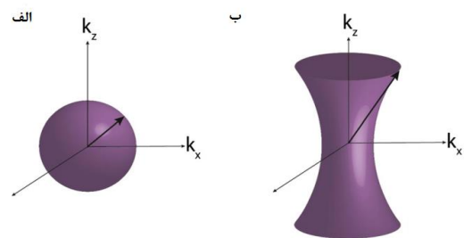
شکل ۱: سطح هم فرکانس برای، الف: دی‌الکتریک همسانگرد ب: فرامواد ناهمسانگرد با \varepsilon_{\perp} > 0 و \varepsilon_{\parallel} < 0 [۴].
