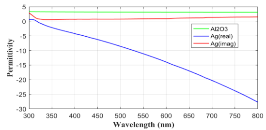
شکل ۵: ضریب گذردهی الکتریکی اجزای سازنده: اکسید آلومینیوم و نقره (بخش حقیقی و موهومی)
