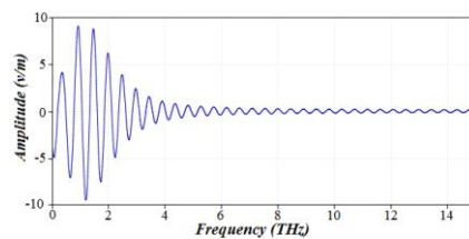
شکل ۸: طیف فرکانسی مربوط به چشمه نوری گاوسی
