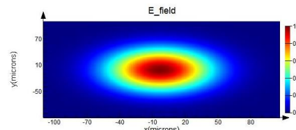
شکل ۳: الگوی دامنه میدان الکتریکی چشمه نوری
