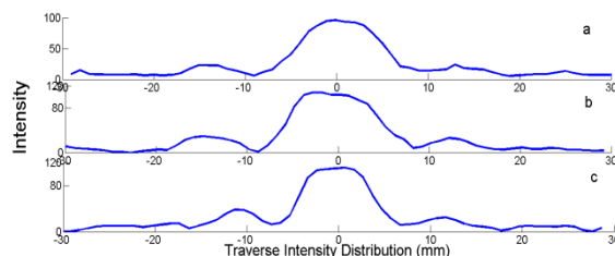
شکل ۱۲: نقاط کانون عدسی شعاع ۷,۵ میلیمتر: a نقطه‌ی کانون در ۶۰۰ میلیمتر، b نقطه‌ی کانون در ۱۰۰۰ میلیمتر
