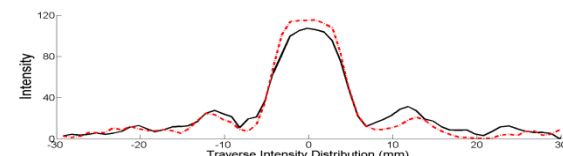
شکل ۱۷: توزیع شدت در نقاط کانون عدسی: نمودار قرمز توزیع شدت در فاصله‌ی ۶۰۰ میلیمتر و نمودار مشکی مربوط به توزیع شدت در فاصله ۱۰۰۰ میلیمتر
