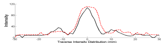
شکل ۱۵: توزیع شدت در نقاط کانون عدسی: نمودار قرمز توزیع شدت در فاصله‌ی ۶۰۰ میلیمتر و نمودار مشکی مربوط به توزیع شدت در فاصله ۱۰۰۰ میلیمتر
