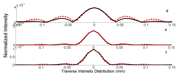
شکل ۷: توزیع شدت در نقاط کانون هر سه عدسی: d شعاع ۷,۵ mm e. شعاع ۸,۵ mm f, شعاع ۱۰,۵ میلیمتر. نمودار قرمز توزیع شدت در کانون ۶۰۰ میلیمتر و نمودار مشکی مربوط به توزیع شدت در کانون ۱۰۰۰ میلیمتر است.
