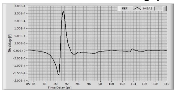
شکل ۱: سیگنال زمانی تراهرتز
