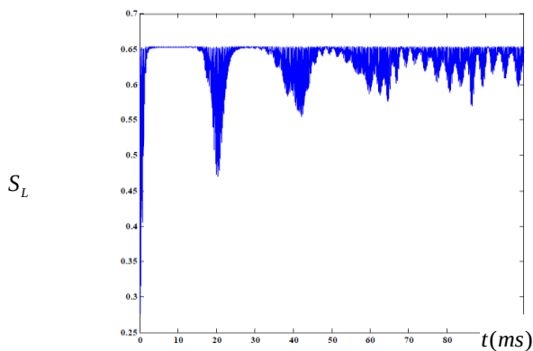
شکل ۴: آنتروپی خطی برای یون به دام افتاده نوع نردبانی. سایر پارامترها عبارتند از f(n_j) = \sqrt{n_j} ، n_1 = n_2 = 10 ، m = 4 ، g = 10^4 \text{ Hz} و \chi = 10^3 \text{ Hz} .
