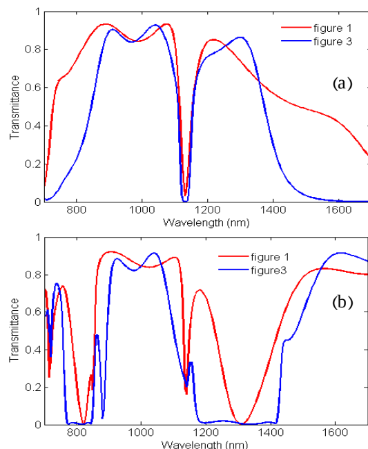
شکل ۴: عبور موجبر شکل‌های ۱ و ۳ به ازای (a) حالت \epsilon_1 = 3.2 ، (b) حالت \epsilon_1 = 5.7 ، h = 200\text{nm} و h = 300\text{nm} .
