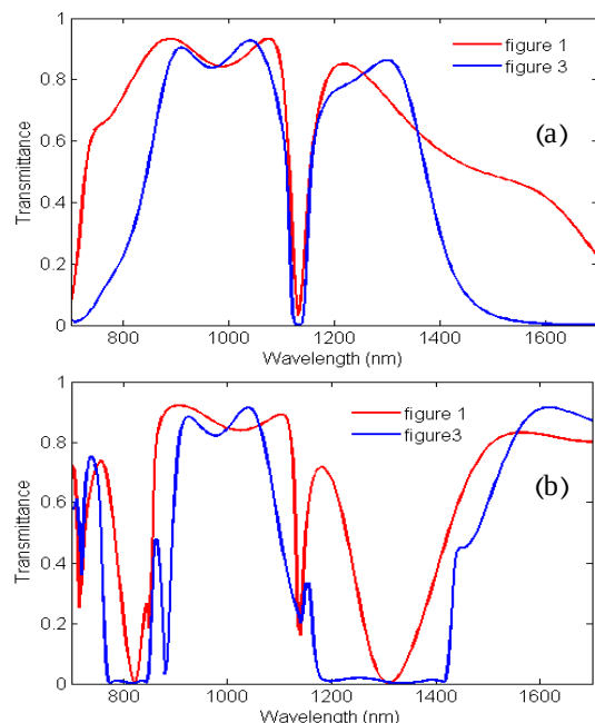
شکل ۴: عبور موجبر شکل‌های ۱ و ۳ به ازای (a) حالت \epsilon_1 = 3.2 ، h = 200 \text{ nm} و (b) حالت \epsilon_1 = 5.7 ، h = 300 \text{ nm} .
