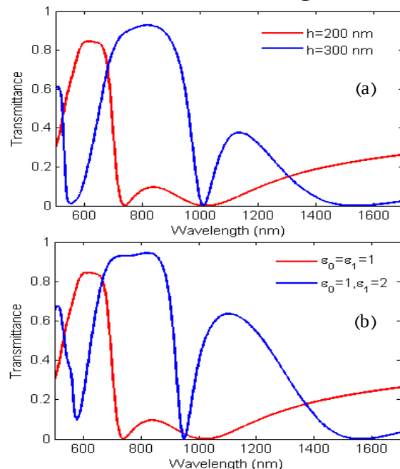
شکل ۲: عبور موجبر شکل ۱ برای (a) ارتفاع‌های مختلف و (b) جنس مختلف ماده داخل شیار.
