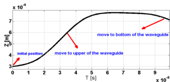
شکل ۶: حرکت نانوذره طلا- دی اکسید تیتانیوم که در مکان اولیه در انتهای موجبر قرار گرفته است.
