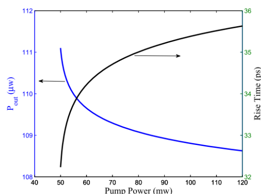
شکل ۳: اثر تغییرات توان پمپ روی الف) توان خروجی، و ب) زمان بازایی جمعیت حامل ها در تراز N_3 ، با توان پروب ۱۰ میلی وات و عرض پالس ۵ پیکوثانیه
