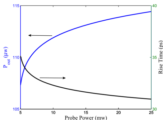
شکل ۴: اثر تغییرات توان پروب روی الف) توان خروجی، و ب) زمان بازایی جمعیت حامل ها در تراز N_3 ، به ازای توان پمپ ۱۰۰ میلی وات و عرض پالس ۵ پیکوثانیه
