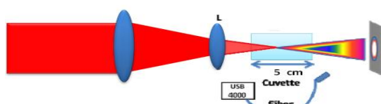
شکل ۱: نمایش طرح وار چیدمان آزمایشگاهی برای تولید ابرپیوستار
