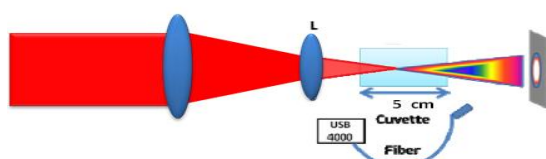
شکل ۱: نمایش طرح وار چیدمان آزمایشگاهی برای تولید ابرپیوستار
