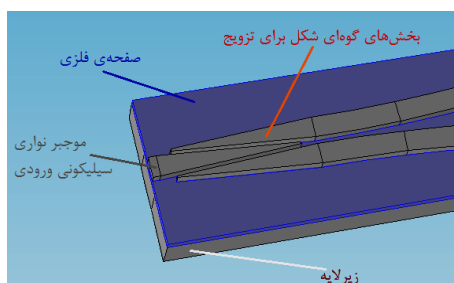
شکل ۱- ساختار تقسیم‌کننده‌ی توان پلاسمونیک با ۳ بخش گوه‌ای شکل
