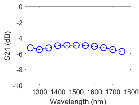
شکل ۷- طیف S_{21} تقسیم‌کننده با نوارهای خروجی پلیمری
