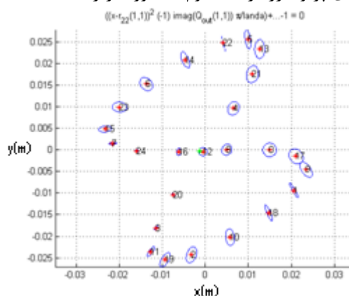
شکل ۴: لکه های پرتو لیزر در آینه ی دوم با مقادیر رابطه ی (۱۶)
