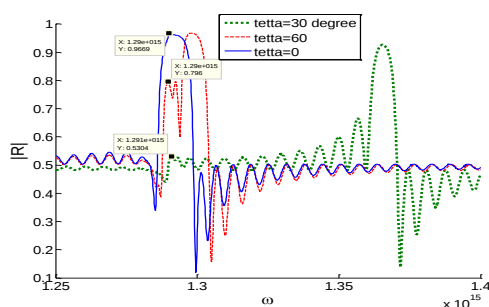
شکل ۲: بازتابندگی چاه کوانتومی InGaAs/GaAs دوره ی زاویه تابش \theta=0 درجه (نمودار آبی)، \theta=30 (قرمز نقطه چین) و \theta=60 (نمودار سبز خط چین) می باشد.
