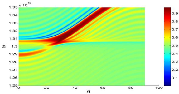
شکل ۵: نواحی قرمز، گاف باند بلور فوتونی متشکل از نیم رساناهای چاه کوانتومی InGaAs/InAs که تحت پالس دماش قرار دارد، می‌باشد.
