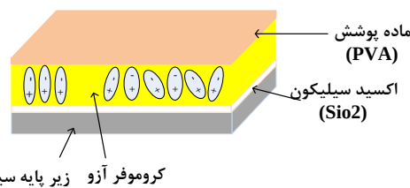
شکل ۳: شکل لایه‌های فیلم نازک پلیمر برای ساخت موجبر مایخزنر.
