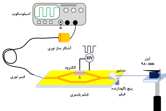
شکل ۴- چیدمان آزمایشگاهی برای مدولاسیون الکترو-اپتیک و تزویج نور لیزر ۹۸۰ نانومتر همزمان با اعمال ولتاژ ثابت به مایخزنر.
