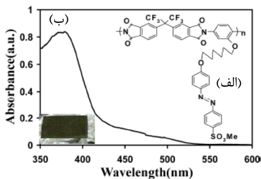
شکل ۲: (الف) ساختار شیمیایی رنگدانه ی آزو متصل شده به پلیمر، (ب) طیف جذب ماده استفاده شده.
