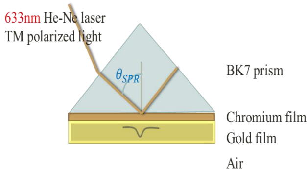
شکل ۱: هندسه ی کرشن در چیدمان تجربی
