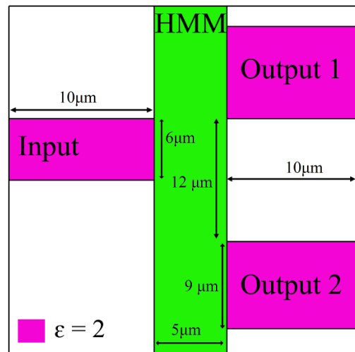
شکل ۵: ساختار پیشنهادی برای y-branch
