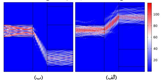
شکل ۷: نحوه عملکرد y-branch به ازای پتانسیل شیمیایی (الف) 0.4 \text{ eV} و (ب) 0.5 \text{ eV}
