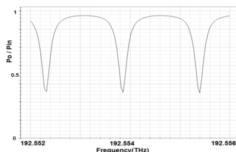
شکل ۸ پاسخ فرکانسی تشدیدگر با شعاع ۳cm- ضریب تزویج ۰,۰۵db- تلفات ۰,۰۰۵db/cm
