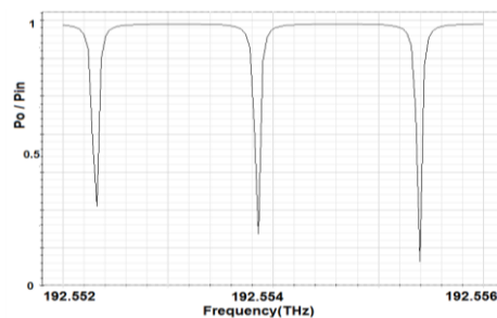
شکل ۷ پاسخ فرکانسی تشدیدگر با شعاع ۳cm- ضریب تزویج ۰,۰۵db- تلفات ۰,۰۰۵db/cm
