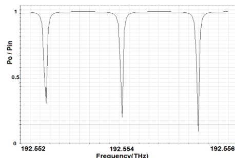
شکل ۹ پاسخ فرکانسی تشدیدگر با شعاع ۳cm- ضریب تزویج ۰,۰۵db- تلفات ۰,۰۰۵db/cm
