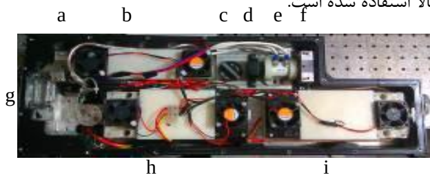
شکل ۴: چیدمان تجربی لیزر نئودیمیم یاق Q-سوئیچ شده (a: آینه جلویی، b: کاواک لیزر، c: تیغه پلاریزور، d: تیغه ربع موج، e: سلول پاکلز، f: آینه عقبی، g: منشور فولد، h: تقویت کننده اول، i: تقویت کننده دوم).
