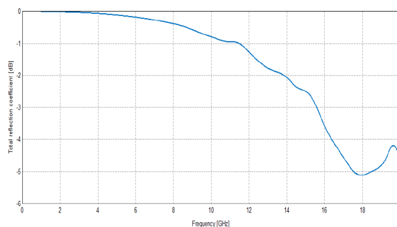
شکل ۵: تلفات انعکاس برای نمونه LZCF با آلایش CNT
