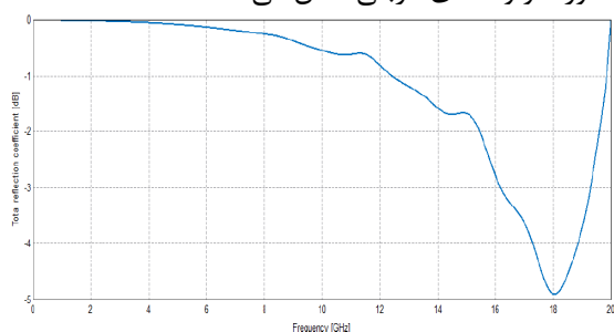
شکل ۴: تلفات انعکاس برای نمونه CNZF با آلایش CNT
