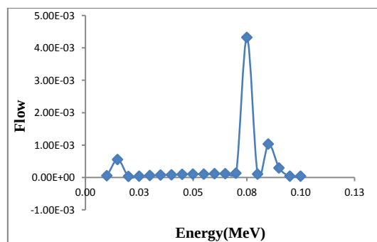
شکل ۵: جریان فوتونی (مشخصه و ترمزی) برای فرود 85^\circ و زوایای خروج ۱۱۵ تا ۱۲۰ درجه.
