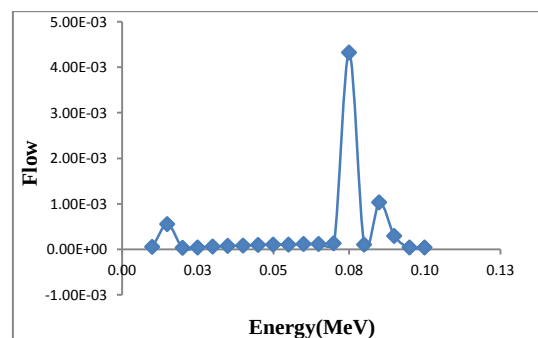
شکل ۵: جریان فوتونی (مشخصه و ترمزی) برای فرود 85^\circ و زوایای خروج 115 تا 120 درجه.
