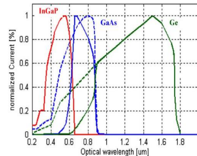
شکل ۵: پاسخ فرکانسی سه سلول به صورت جداگانه
