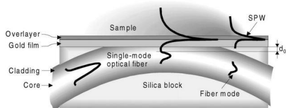
شکل ۱- برانگیختگی پلاریتون پلاسمون سطحی در تار نوری کنار ساییده شده [۳].
