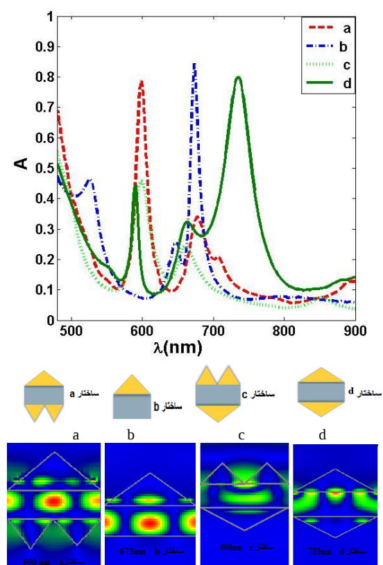
شکل ۱ مقایسه جذب ساختارهای طراحی شده و بررسی توزیع میدان مغناطیسی در طول موج پیک هر یک از ساختارها
